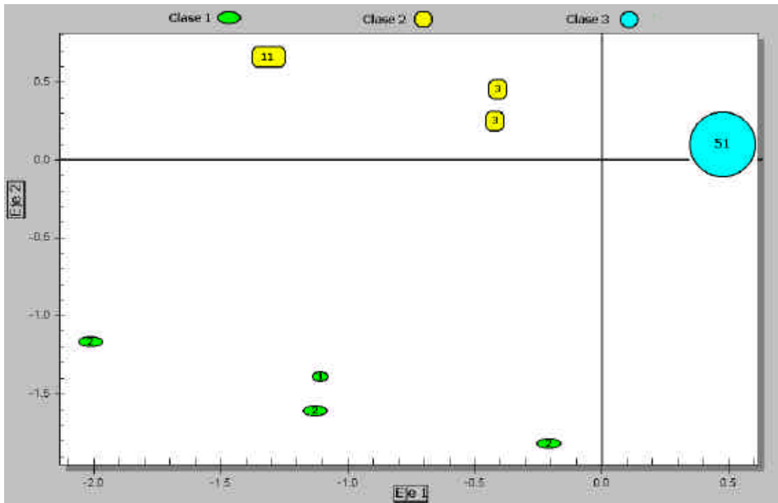
Gráfico 1: Primer Plano Factorial del espacio de individuos correspondiente a la clasificación obtenida para el contexto de descubrimiento.
